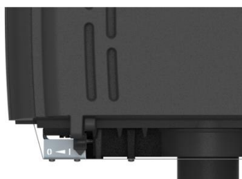
Position d'allumage: Apport d'air et air d'allumage ouvert
